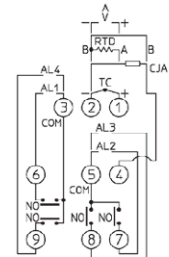
⑩ ⑪ V PWR U (11Pソケット)
