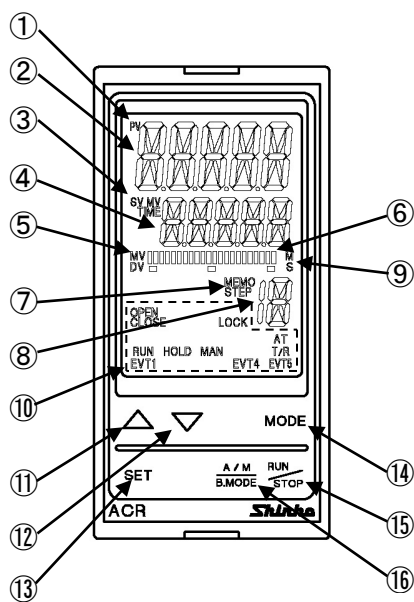
ACR-15A
