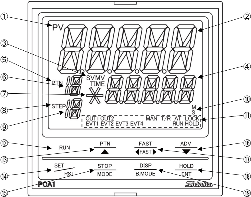
PCA1 正面
