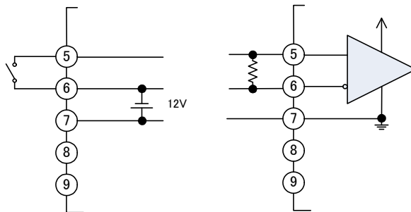
有接点スイッチ [SAFU-1□-□(超スロー パルス変換器)のみ]
