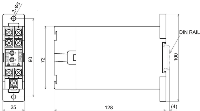
3.1 外形寸法図(単位: mm)
