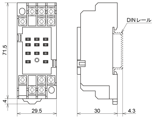
11P ソケット(SGFW)
