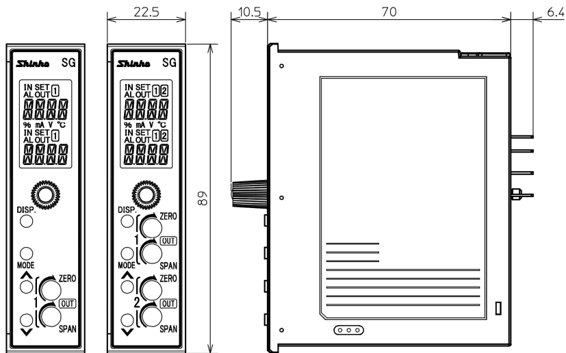
8P ソケット(SGI, SGIL)
