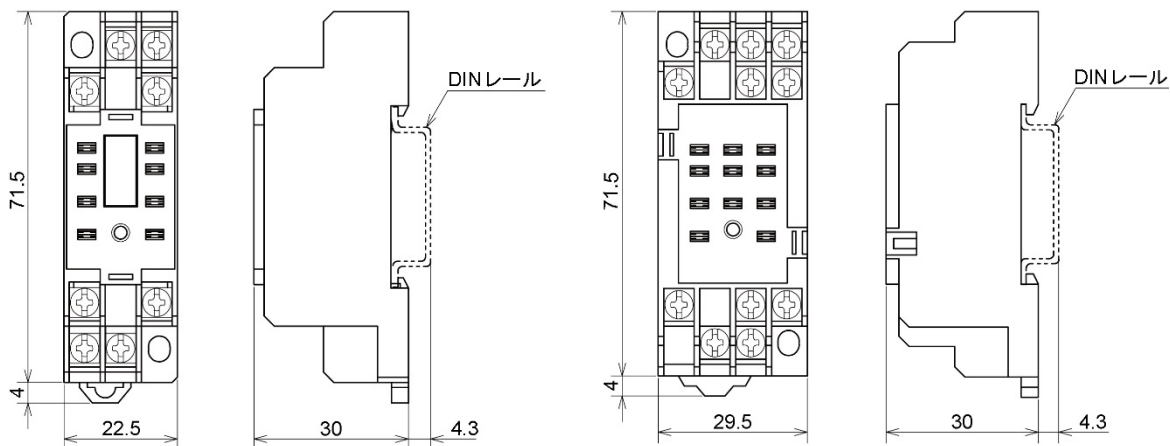
8P ソケット(SGU, SGUL)
