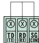
⑥: RS-232C通信機能端子 (オプション)
