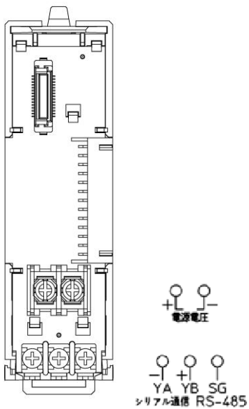
[ベース部]QDM1-□□□□
