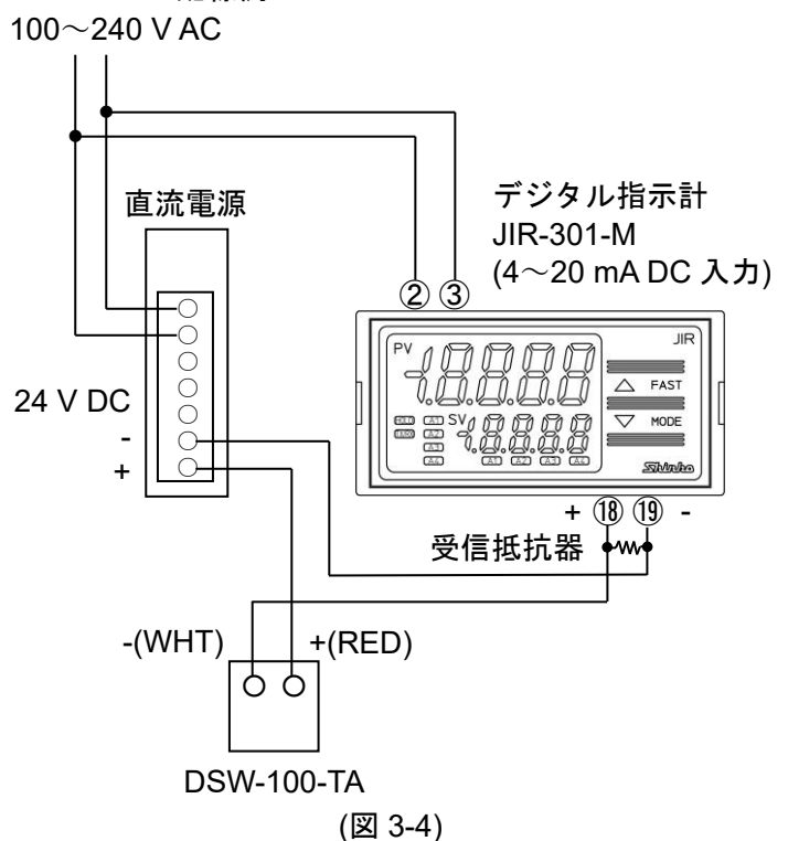
DSW-100-TA 配線例
