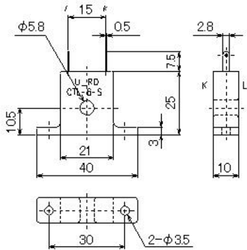
CTL-6-S-H(20 A 用)
