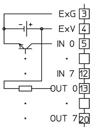
RG-CU-DIO8A (NPN)
