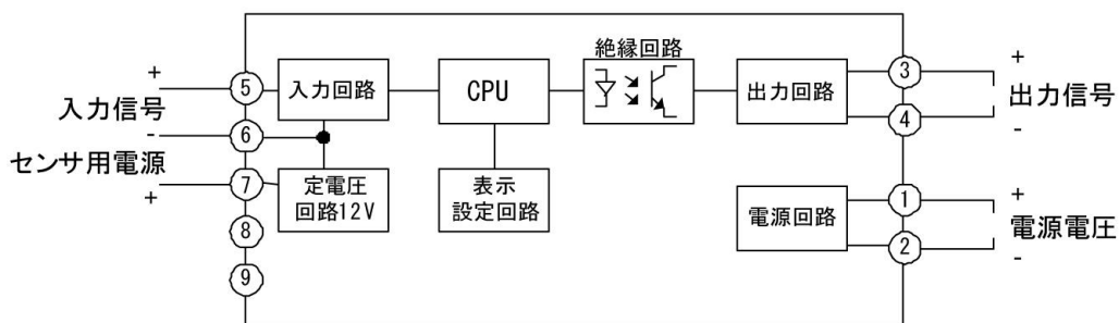
入力接続例
