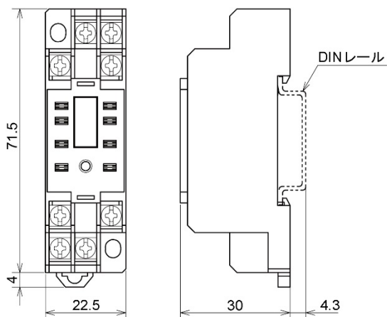
8P ソケット(SGB, SGBL)
