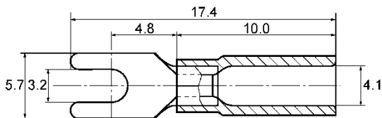
Y形压着端子外形图(单位:mm)
