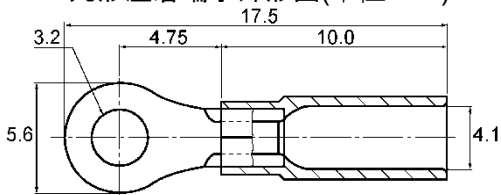
丸形压着端子外形图(单位:mm)
