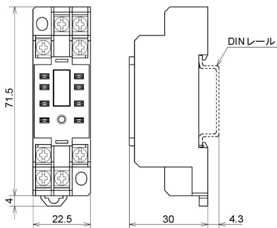
8P ソケット(SGT, SGTL)
